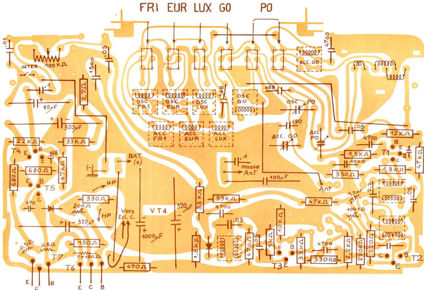
CIRCUIT IMPRIMÉ VU COTÉ CUIVRE
