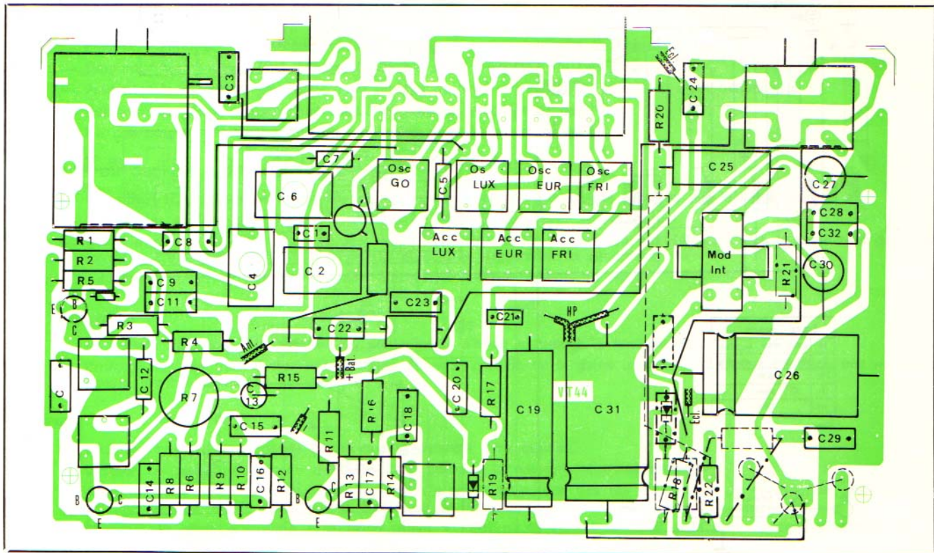
IMPLANTATION CIRCUIT IMPRIME VU COTE CUIVRE
