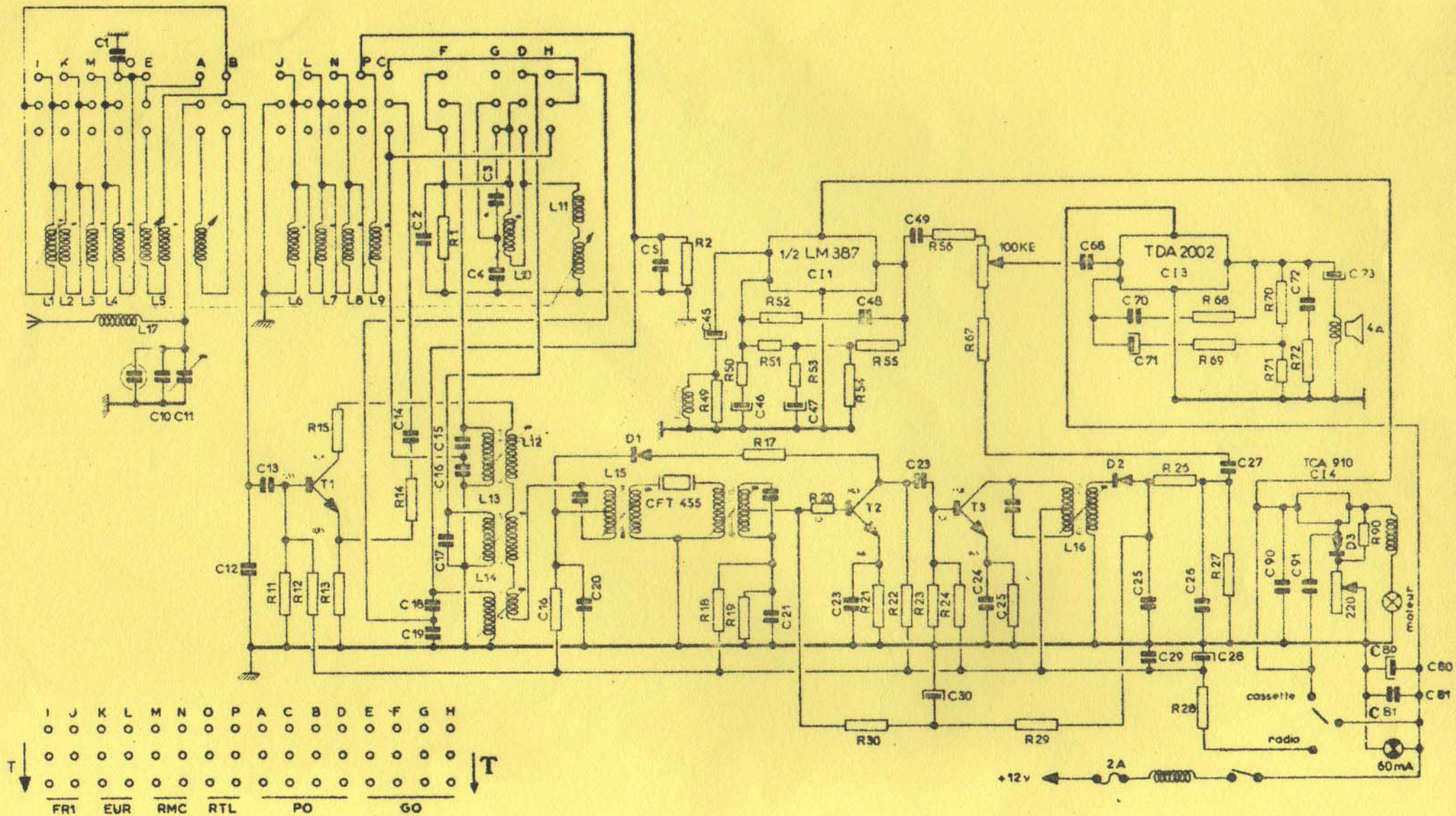
SCHEMA THEORIQUE AUTO-CASSETTE MONO PO GO. 4 Pré-réglés TOURAINE
