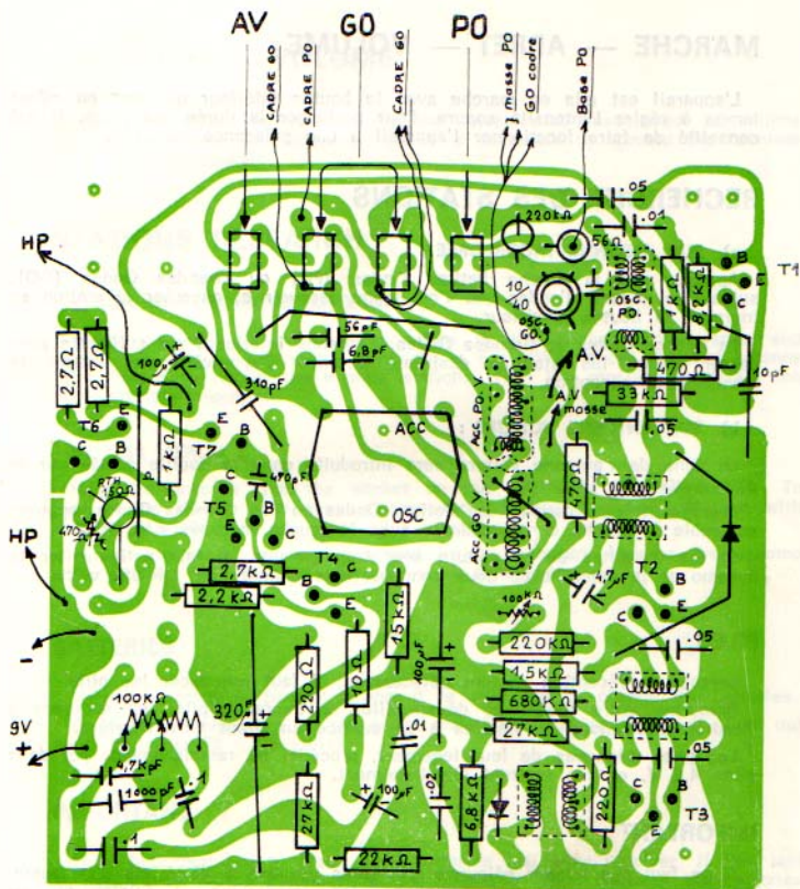
CIRCUIT IMPRIME VU COTE CUIVRE
